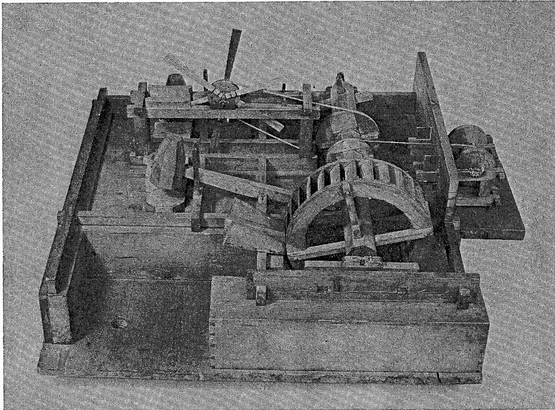
Modell av "Norrländsk Bråk- och Skäkt-Machin at med vattendrift bråka, skäkta och bereda Linet". Nr 255 i Kongl. Modellkammarens inventarium, tryckt i Extraposten 1795. — Tekniska Muséet 1.335.
