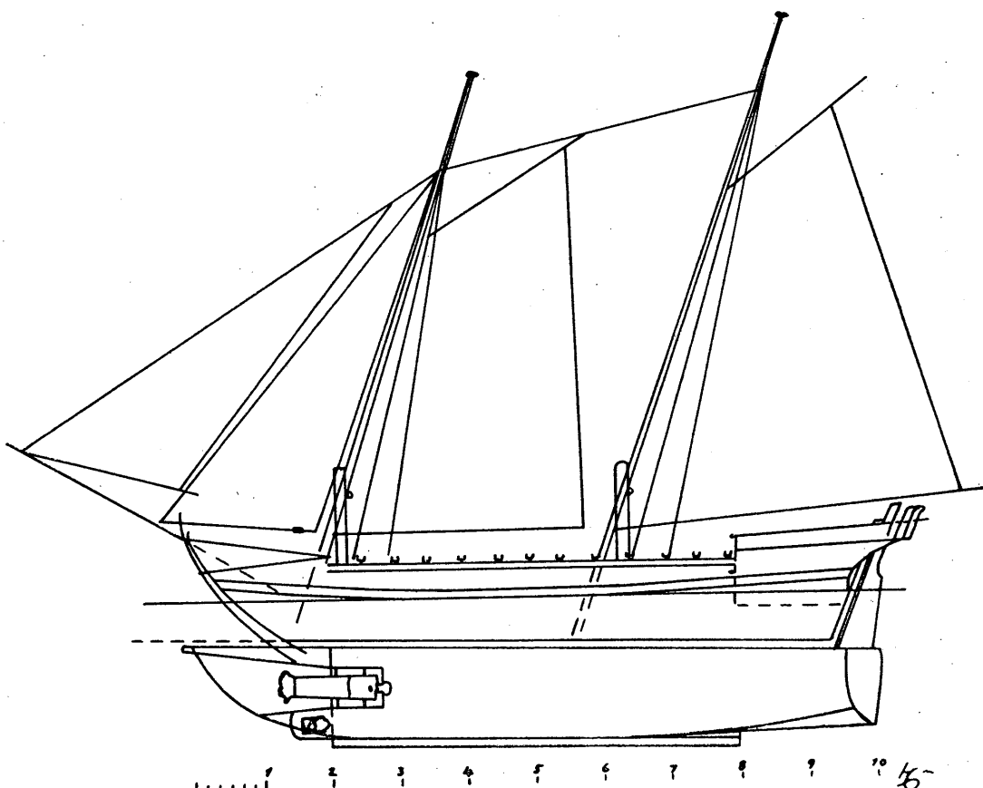
Teckning av kanonslup av skärgårdsflottans typ bestyckad med 2 kanoner och 2 nickor samt plats för 12 par roddare. Efter en teckning av eventuellt S. Bennets hand. Originalen i B. S. A.
